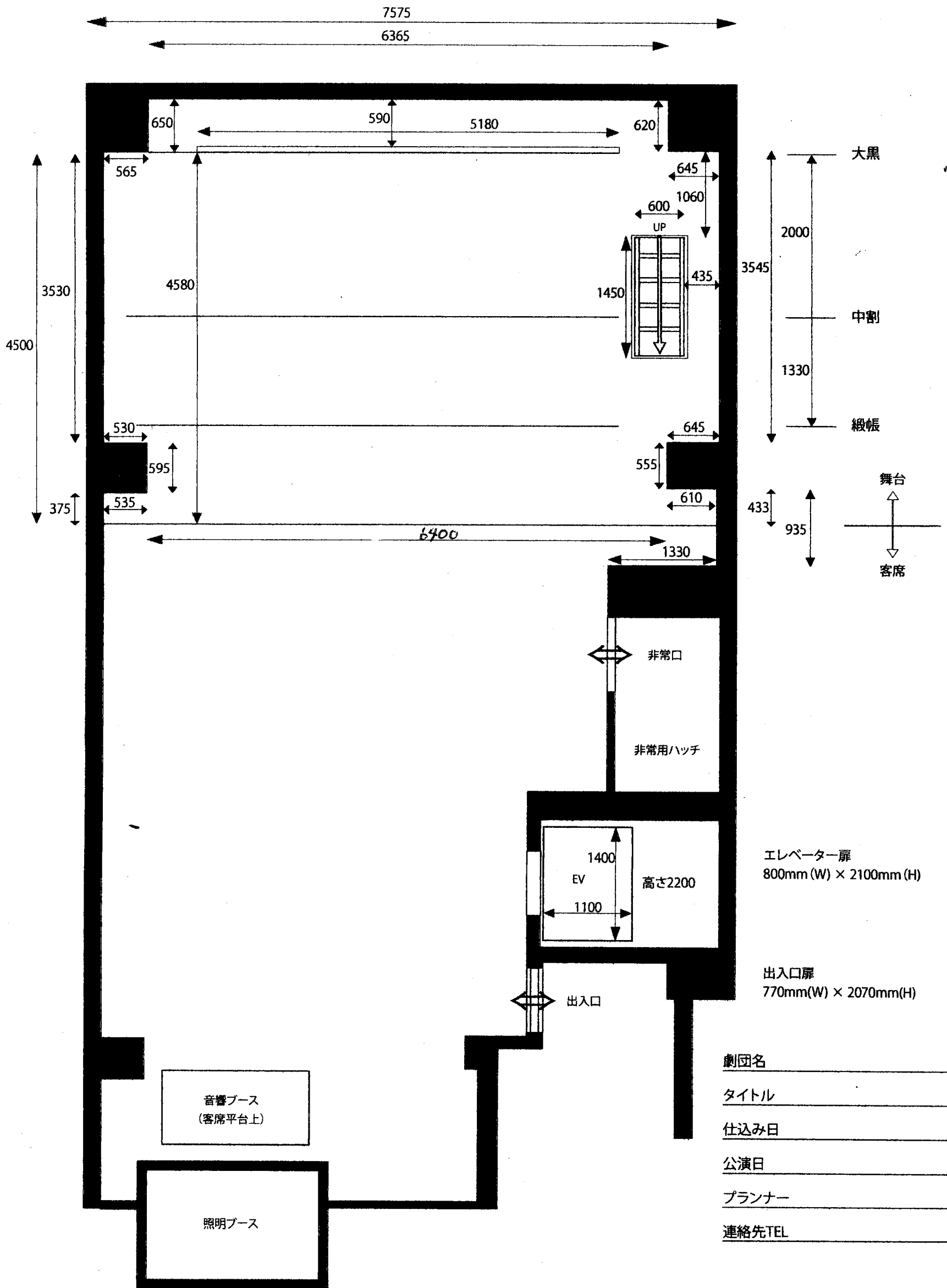
平面図 (縮尺1/50)
